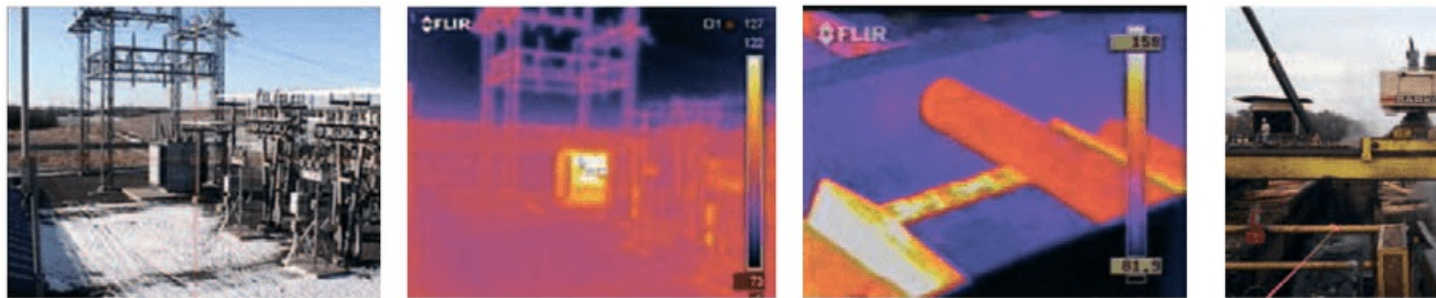
Цифровое фото и ИК-изображение подстанции с перегретым трансформатором
