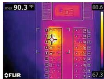
Область с горячим участком указывает на работающий плавкий предохранитель
